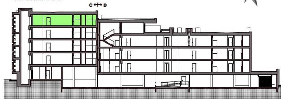
ŘEZ OBJEKTY C+D
