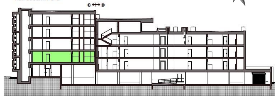
ŘEZ OBJEKTU C+D
