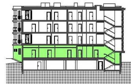
ŘEZ OBJEKTEM A-A
